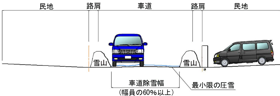
図4-1.8 除雪イメージ(生活道路)
