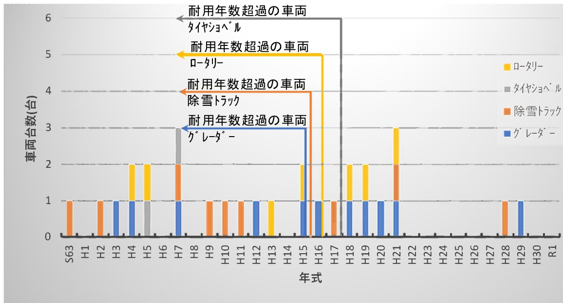
図 4-1.4 除雪機械の年式
