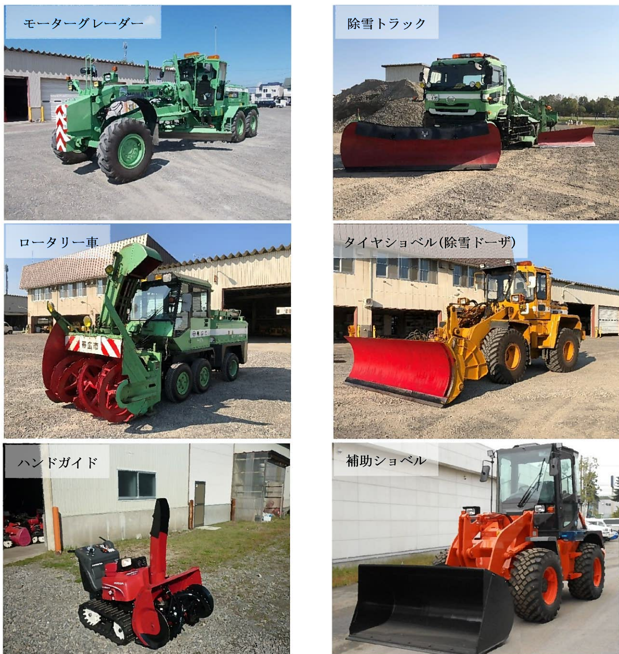
図4-1.3 除雪機械写真
